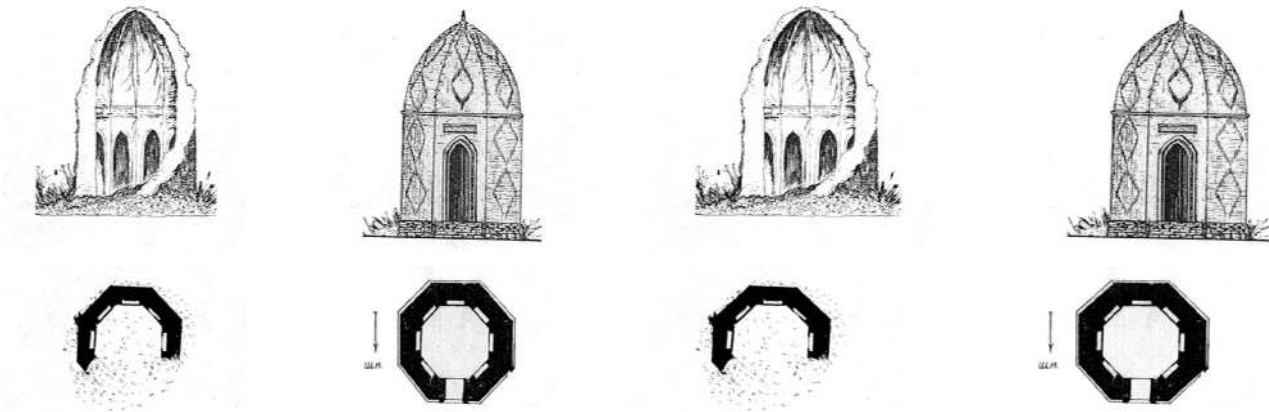
Şəkil 3. Cəlil türbəsinin naturadan çəkilmiş cizgiləri və bərpa layihəsi. Abidənin ölçü işləri, rəsmləri və bərpa layihəsi Rizvan Qarabağlıdır. 1991-ci il
