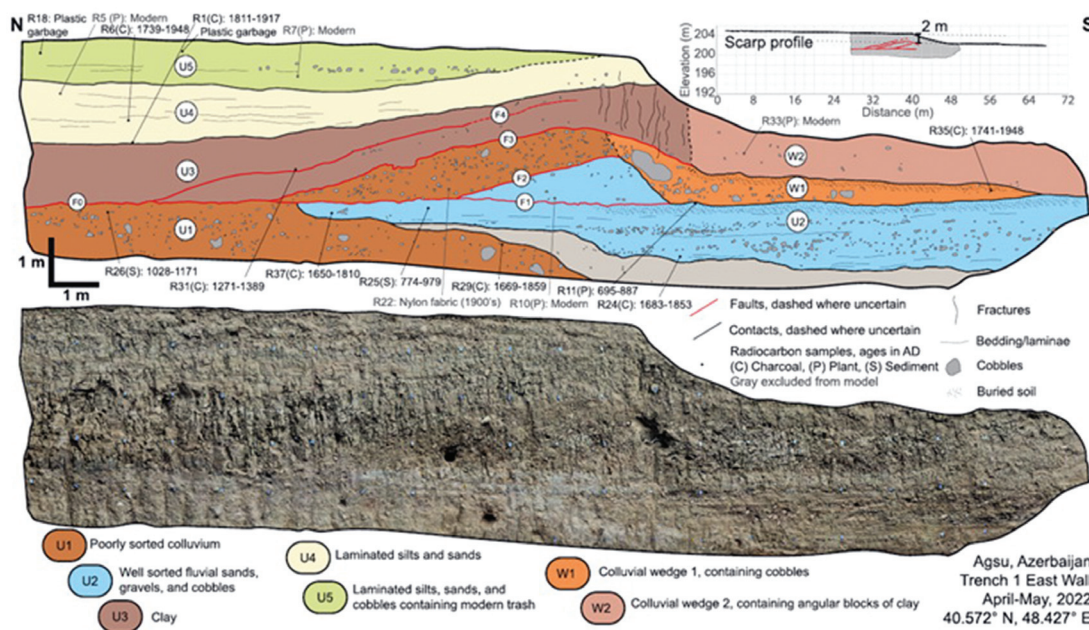
Рис. 2: Геологический разрез, полученный по данным траншеи, раскопанной в 2022 г. в районе Агсу.
