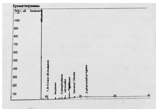
Şəkil 2. Ruta graveolens L.- Ətirli sədo növündən alınan efir yağının xromotoqrafiyası
