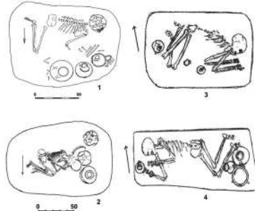
Son Tunc-İlk dəmir (1, 2) və Antik (3, 4) dövrlərinə aid torpaq qəbirləri
