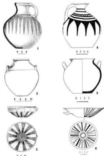
Son Tunc-İlk dəmir (1, 2, 3) və Antik (4, 5, 6) dövrlərinə aid saxsı qabların müqayisəsi
